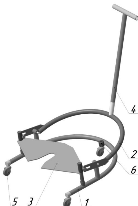
Рисунок 4 – Тележка подкатная
