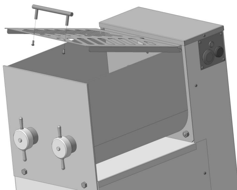
Рисунок – 5 Машина МТ-15М-2(МТ-30)
